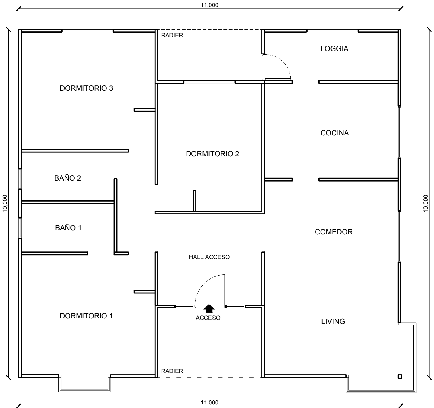
PLANO DE DISTRIBUCIÓN CASA MODELO DON RAÚL 100m²
